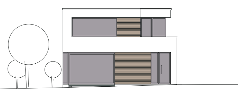
Ansicht Nord | Elevation North
