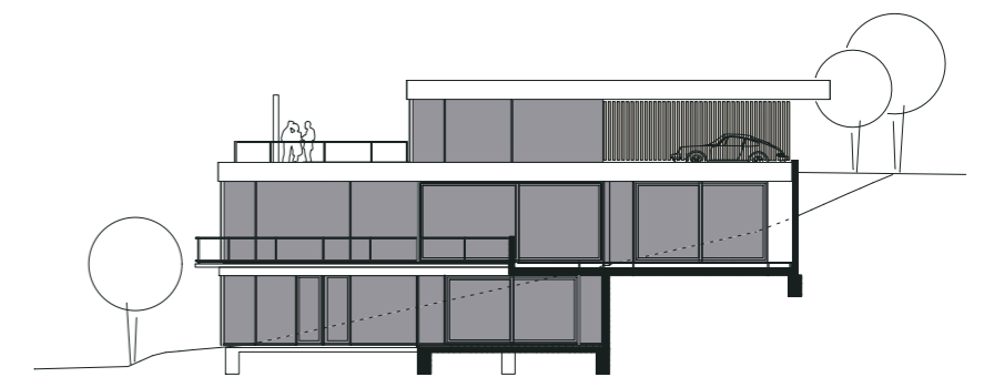
Ansicht Süd | Elevation South
